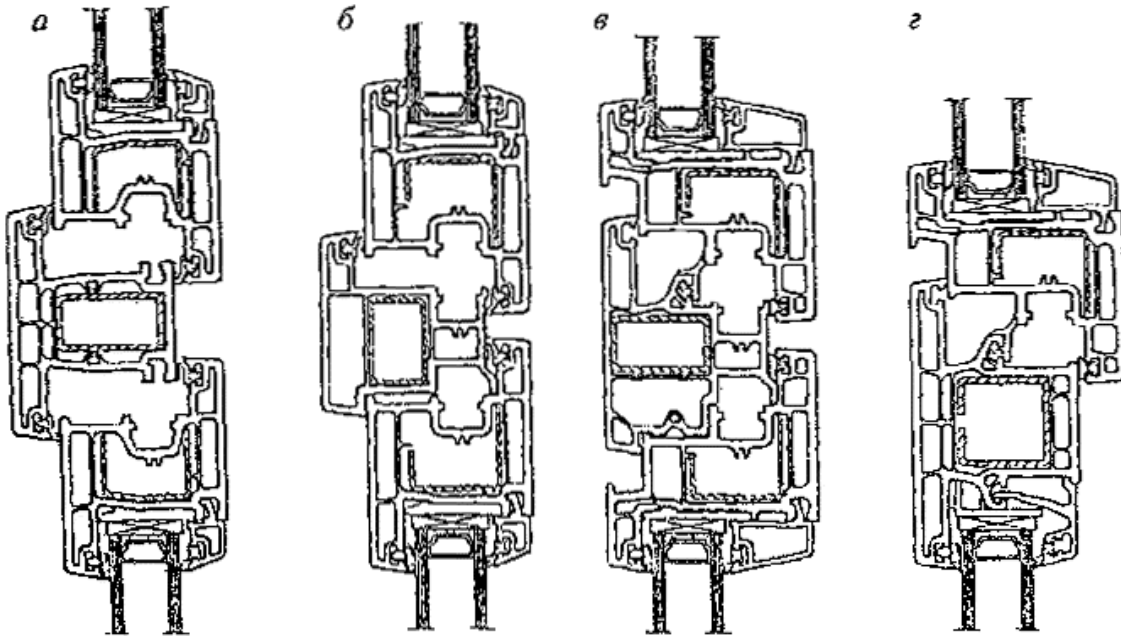
а - импостный притвор оконной системы с наружным и внутренним уплотнениями; б - штапелевой (безимпостный) притвор оконной системы с наружным и внутренним уплотнениями; в - штапелевой (безимпостный) притвор оконной системы со средним и внутренним уплотнениями; г - импостный притвор неоткрывающихся и открывающихся элементов оконной системы со средним и внутренним уплотнениями
