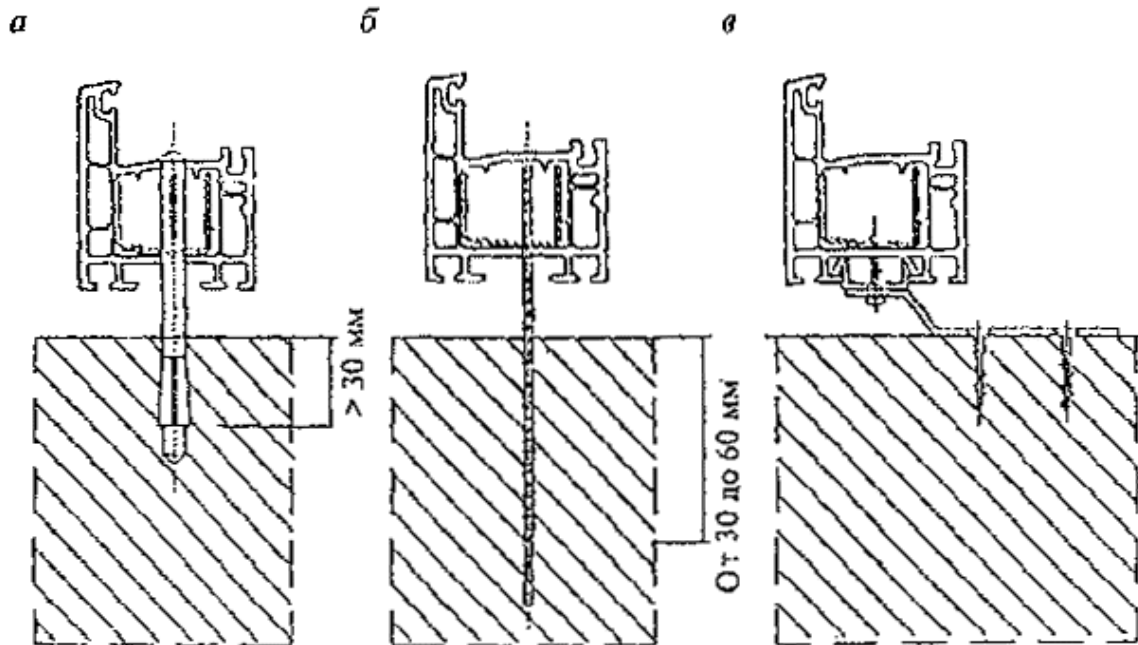
a - узел крепления монтажным дюбелем; б - узел крепления строительным шурупом; в - узел крепления при помощи анкерной пластины
